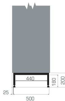
Beine mit einstellbaren Fußschrauben.
