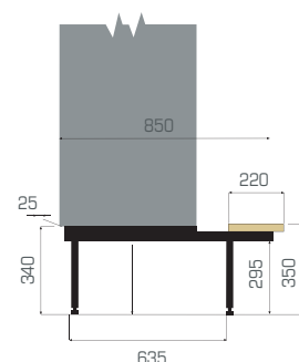
Bankuntergestell für Einzelreihe mit Laminatsitz und einstellbaren Fußschrauben.
