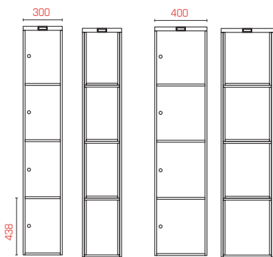
Fjærdedelsskab SFXSH304 og SFXSH404
