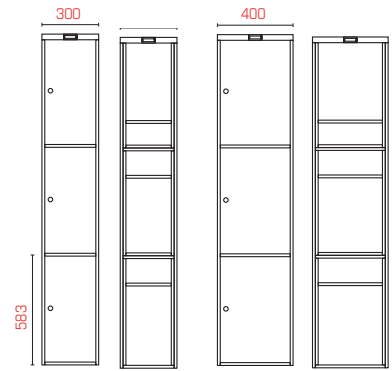
Tredjedelsskab SFXSH303* og SFXSH403*
