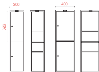
Halvskab SFXSM302* og SFXSM402*
