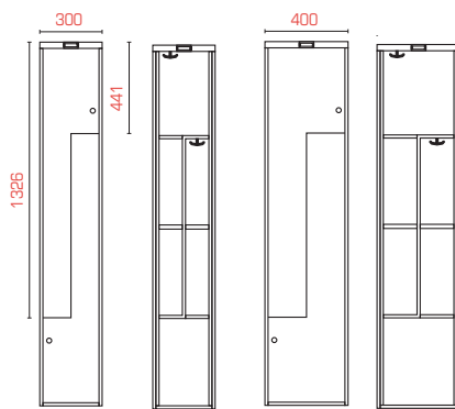
Z-skab SFXSH3Z2 og SFXSH4Z2
