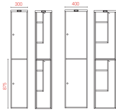
Halvskab SFXSH302* og SFXSH402*
