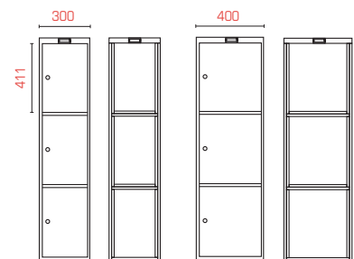
Tredjedelsskab SFXSM303 og SFXSM403
