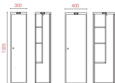
Helskab SFXSM301** og SFXSM401**
