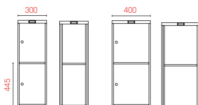
Halvskab SFXSL302 og SFXSL402
