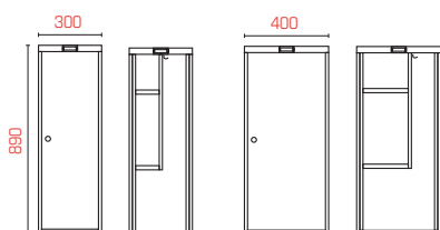
Helskab SFXSL301* og SFXSL401*
