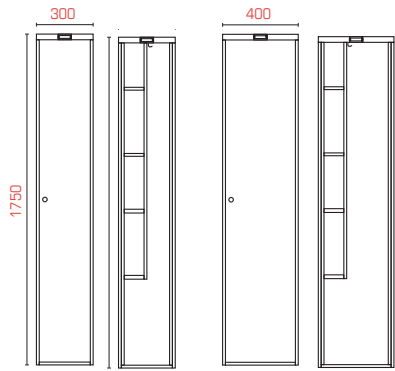
Helskab SFXSH301** og SFXSH401**
