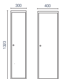
Højskab SFXM301 og SFXM401
