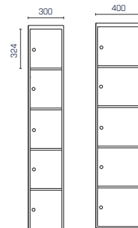
Femdelt skab SFXH305 og SFXH405
