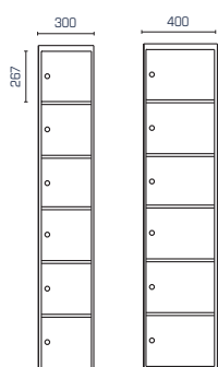
Seksdelt skab SFXH306 og SFXH406
