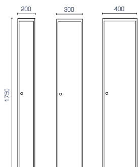
Højskab SFXH201 SFXH301 og SFXH401
