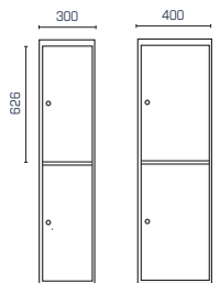
Lavt skab SFXM302 og SFXM402
