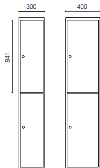
Lavt skab SFXH302 og SFXH402
