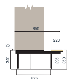
Bænkstativ til enkelttrække med laminatsæde og justerbare stilleskruer.
