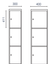
Tredelt skab SFXM303 og SFXM403
