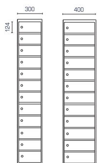
Tolvdelt skab SFXH312 og SFXH412
