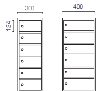
Seksdelt skab SFXL306 og SFXL406
