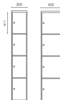
Firdelt skab SFXH304 og SFXH404
