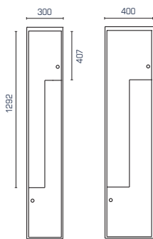
Z-skab SFXH3Z0 og SFXH4Z0
